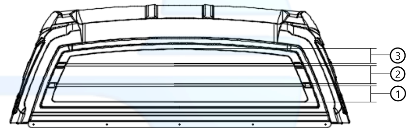
전면 유리 ASSY -①74mm, ②91mm, ③71mm
