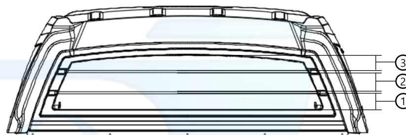
전면 유리 ASSY -①74mm, ②91mm, ③71mm
