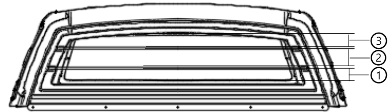
전면 유리 ASSY -①74mm, ②91mm, ③71mm
