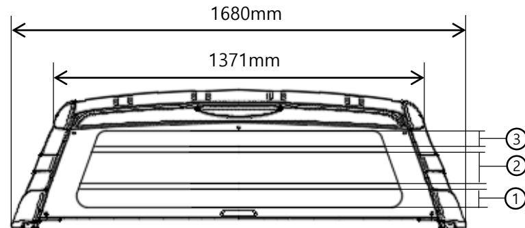
하드탑 도어-①70mm, ②126mm, ③94mm
